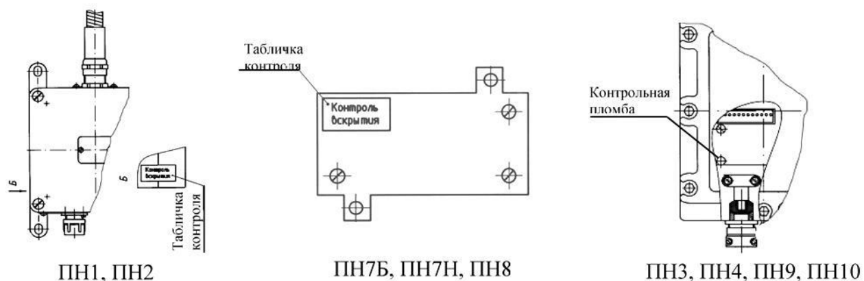
Рис.1 - Схема расположения мест пломбировки и табличек контроля вскрытия
